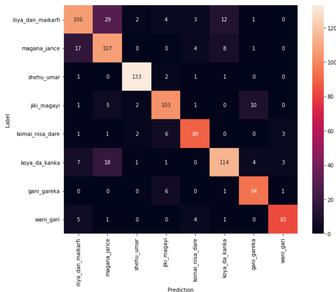
Fig. 8. Confusion Matrix.
